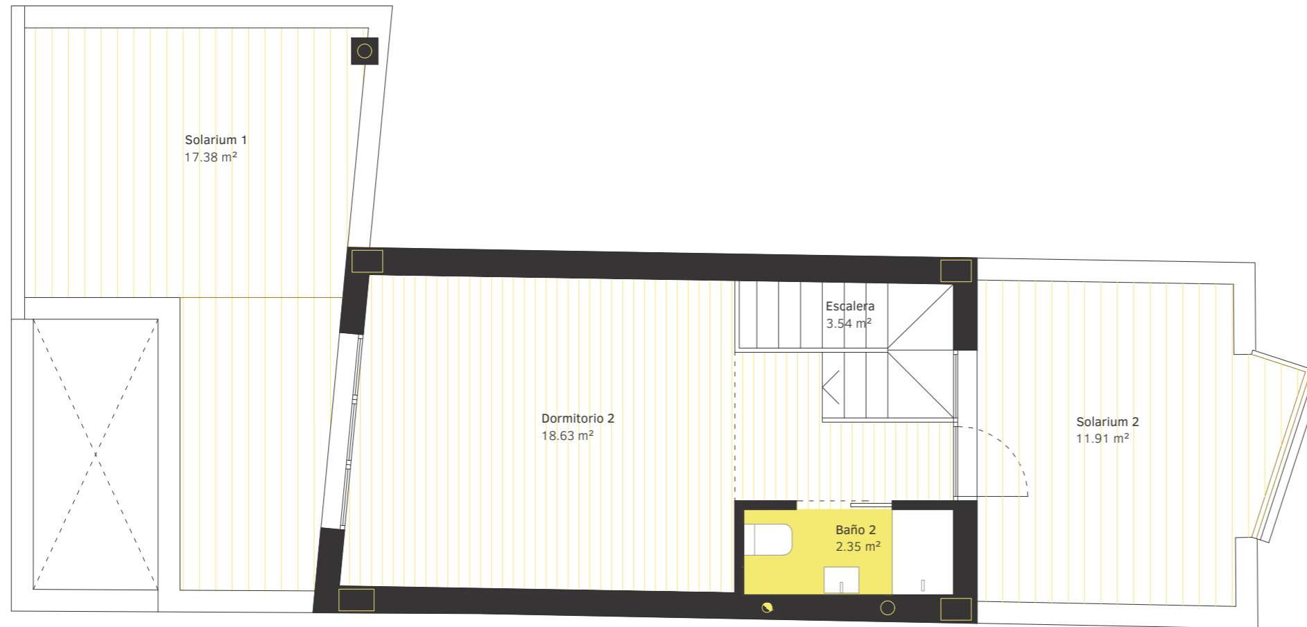
PLANTA ÁTICO
