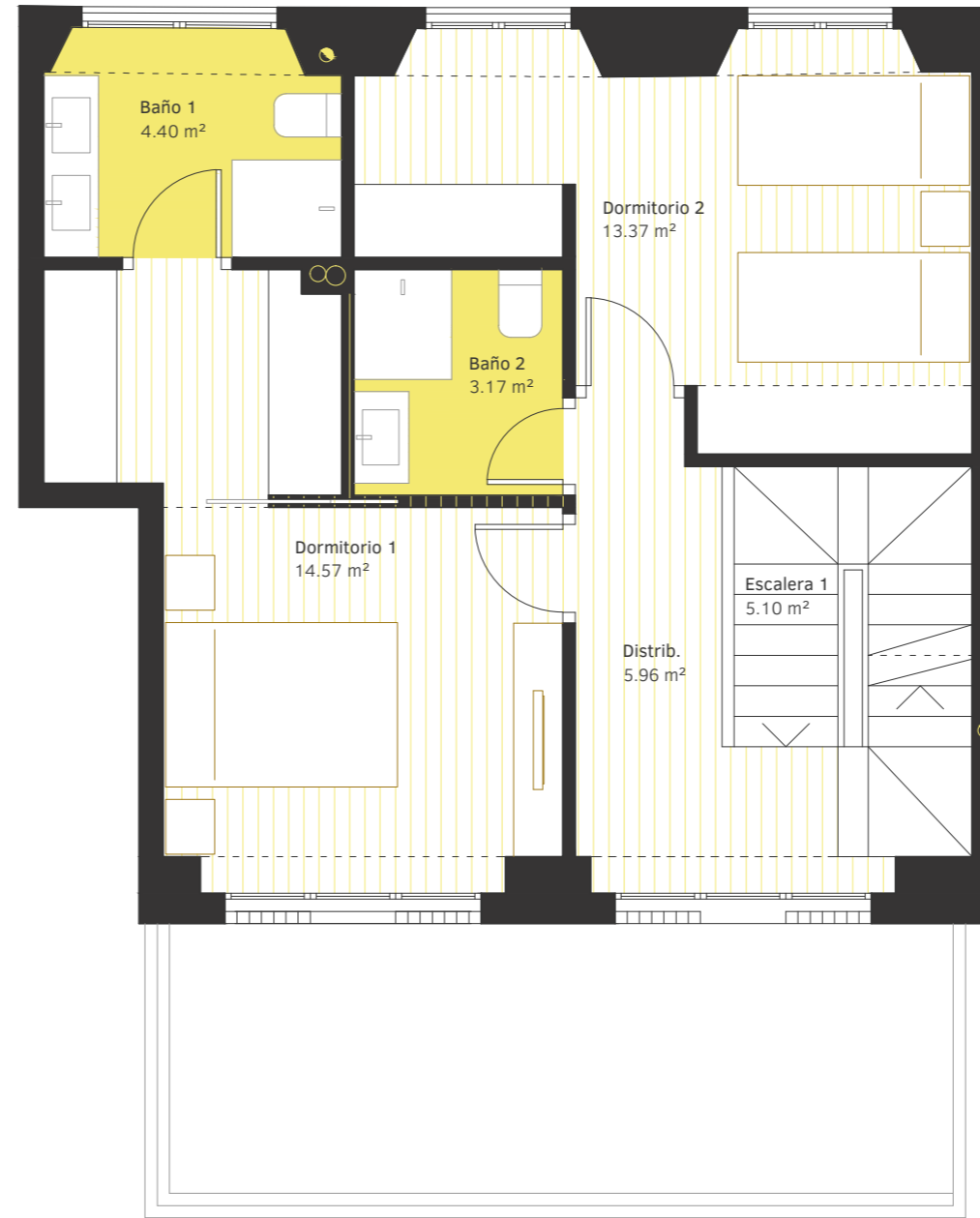
PLANTA PRIMERA
